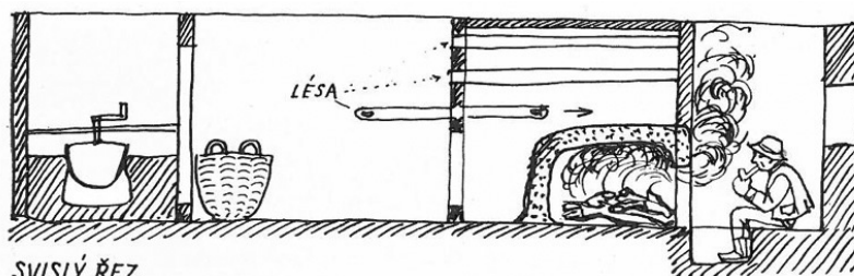
SVISLÝ ŘEZ
